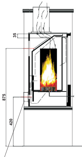
Externe Verbrennungsluftstutzen
