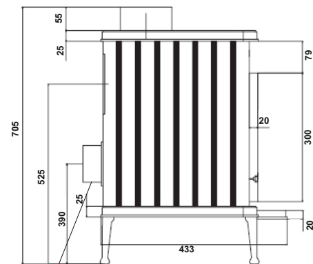
Externer Verbrennungsluftstutzen
