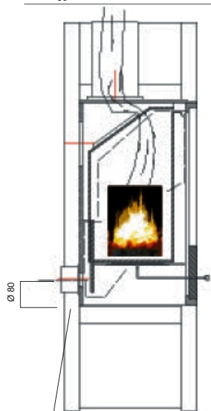
Externe luchttoevoer
