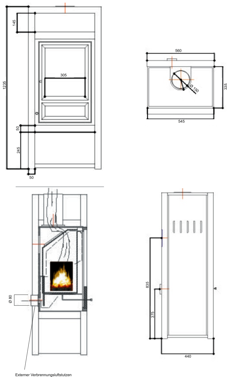
Externer Verbrennungsluftstutzen
