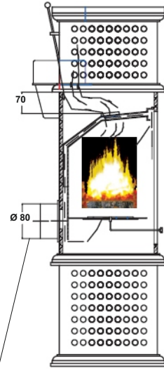
Externer Verbrennungsluftstutzen
